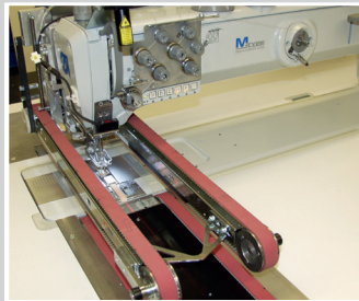
Zusatztransport klein Zusatztransport für gerade Nähte montiert direkt an der Nähma- schine
