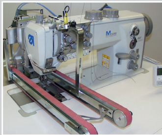
Zusatztransport klein, an einer Zweinadel-Stepstichmaschine
