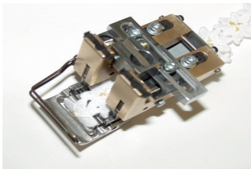
Zick-Zack-Nähfuß mit einem Überstich von 10 mm Art.Nr: MK_94911
