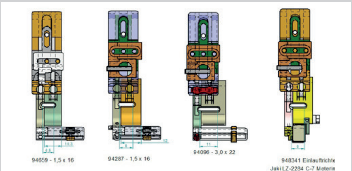
Zick-Zack-Ausgleichsnähfüße zum Gummilitze an- und übernähen. Litzenführung an linker Sohle befestigt
