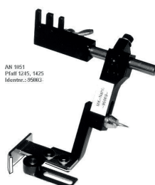
Hochschwenkbarer Anschlag für Leder. Für alle gängigen Nähmaschinenfabrikate
