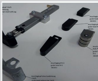
Pneumatischer Stoffkantenanschlag rechts der Nadel mit Zylinder für zwei Kantenabstände und unterschiedliche Anschlagköpfe
