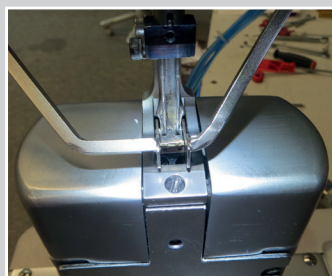
Hochschwenkbarer Stoffkantenanschlag für rechts und links der Nadel.
