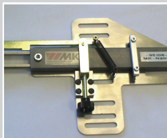
Stoffkantenanschlag auf der Grundplatte mit mehreren Kantenabständen
