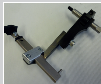
Hochschwenkbarer Stoffkantenanschlag rechts der Nadel, mit Nahtabständen
