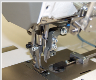
Stanzmesser an einer Flachbett/ Hüpferttransport/Nähmaschine mit pneumatischem Kantenan- schlag
