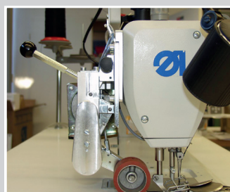
Puller einteilig, 54 mm Zusatztransport für das Nähgut
