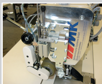
Puller zweiteilig, 54 mm mit Schrittmotor
