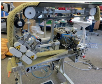
Malerwalzenfertigungs-Automat
