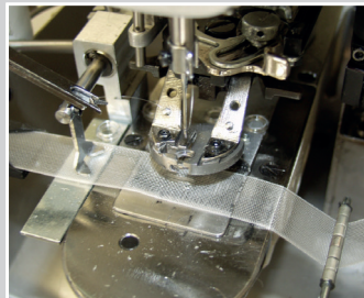
Nähautomat zum Fertigen von Vorhangbändern
