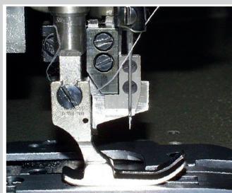
Kantenbeschneidmesser mit Stanzmesser für die Abstufung
