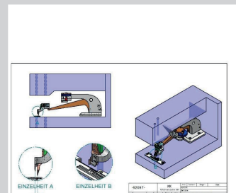
Funktionsbeschreibung des Kantenbeschneidmessers mit daneben montiertem Stanzmesser für die Abstufung
