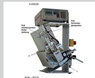
Heizdraht-Schneidegerät 60 mm
