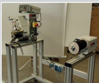
Heizdraht-Schneidegerät 60 mm mit Bandspender auf Rollen
