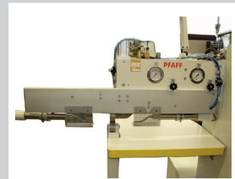
Heißluft mit zwei Heißluftdüsen
