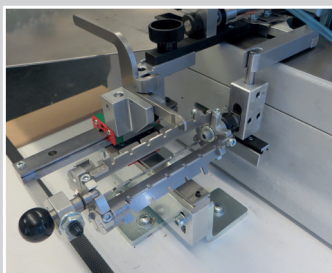
Handindexer für Imitat-Knopflöcher für Einfaden-Kettenstichmaschine
