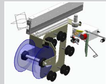
Bandrollenhalter seitlich ausfahrbar mit integrierter Bandüberwachung und Bandsponder für Montage unter der Tischplatte
